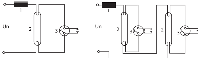
Рисунок 1. Схема подключения
