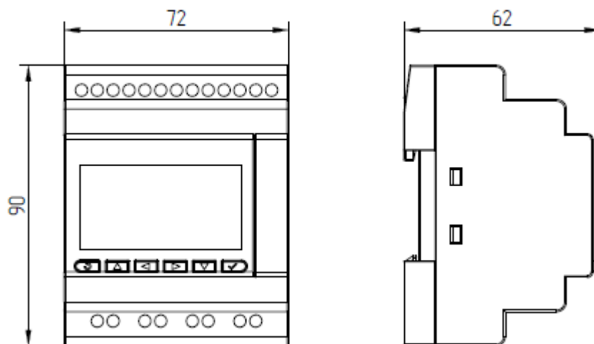
Рисунок 1.1 - Габаритные размеры модуля ЦПУ
