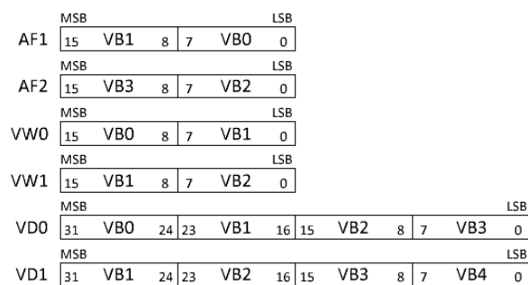
Рисунок 4.83 - Организация структуры памяти
