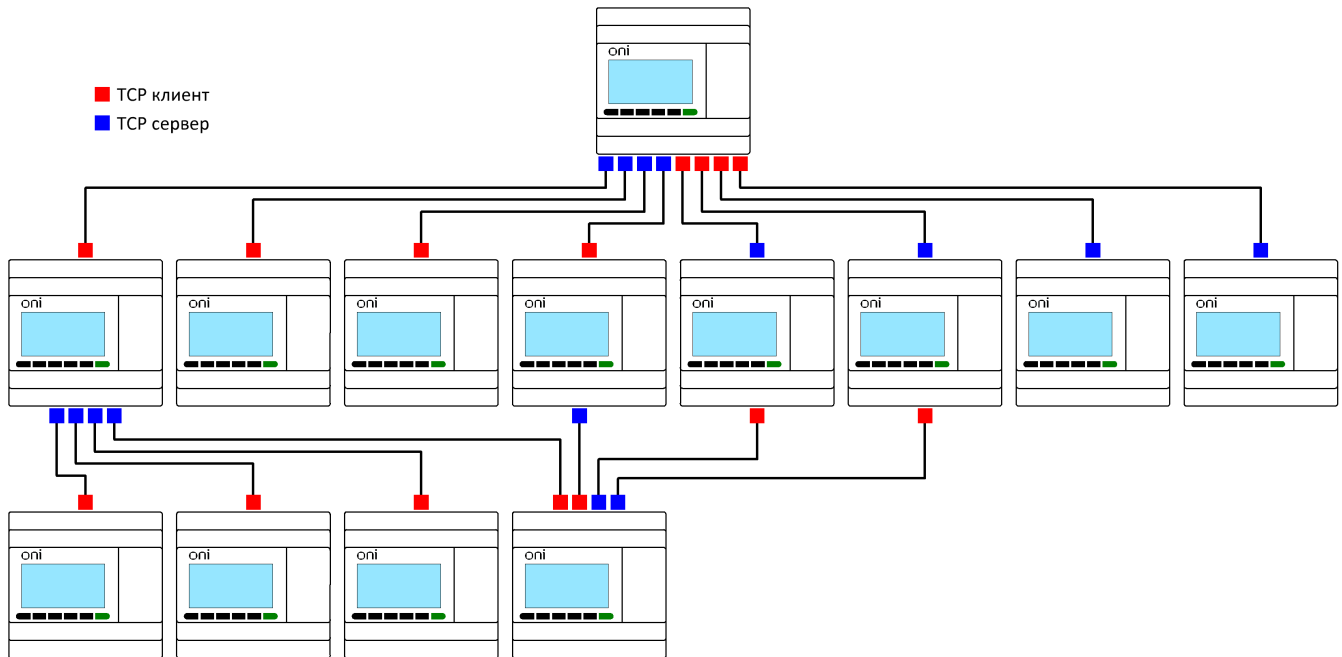
Рисунок 1.45 - Примеры подключения PLC-410
