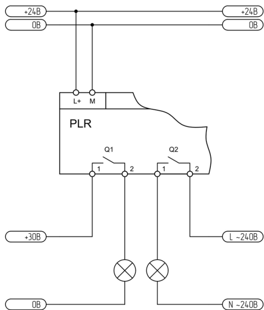
Рисунок 2.14 - Подключение релейного выхода
