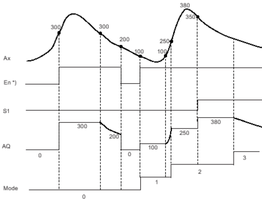
Рисунок 4.164 - Временная диаграмма
