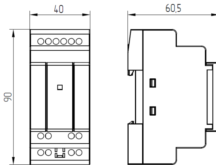
Рисунок 1.13 - Габаритные размеры модуля расширения
