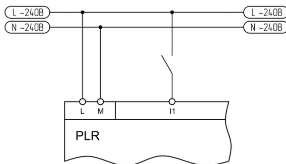
Рисунок 2.18 - Подключение к выходу "сухой контакт"
