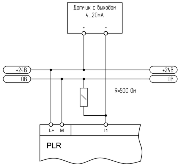
Рисунок 2.7 - Подключение к аналоговому датчику 4-20 мА
