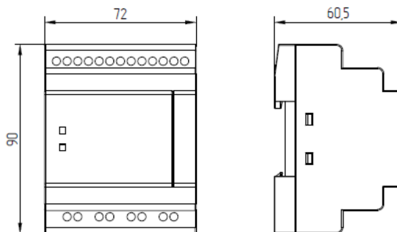
Рисунок 1.2 - Габаритные размеры модуля ЦПУ
