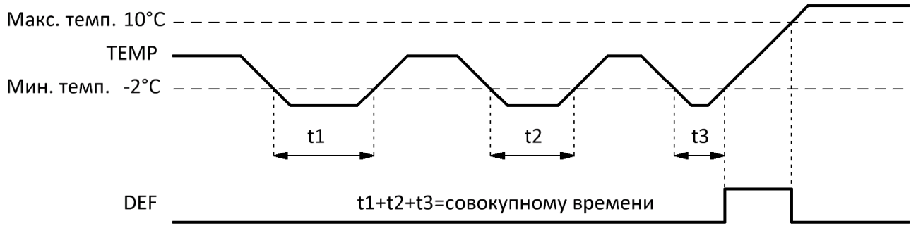
Рисунок 4.207 - Временная диаграмма работы блока
