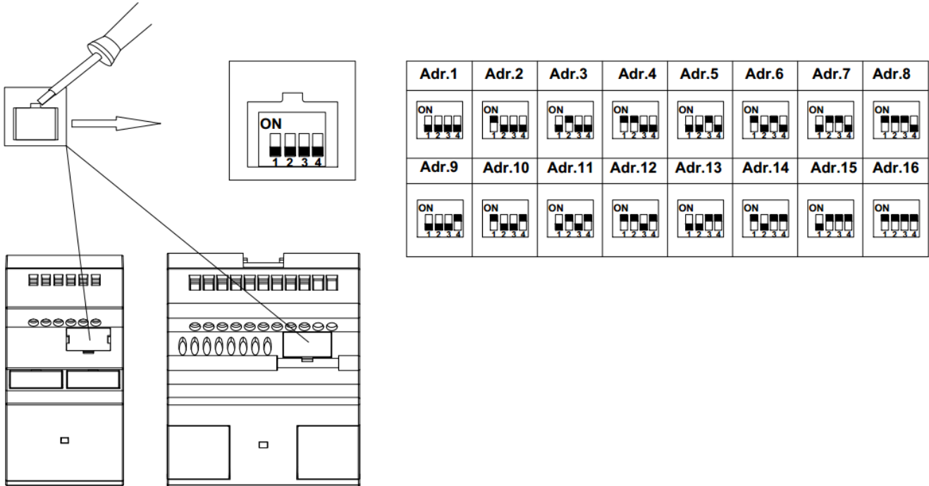
Рисунок 1.26 - Микропереключатели модуля расширения
