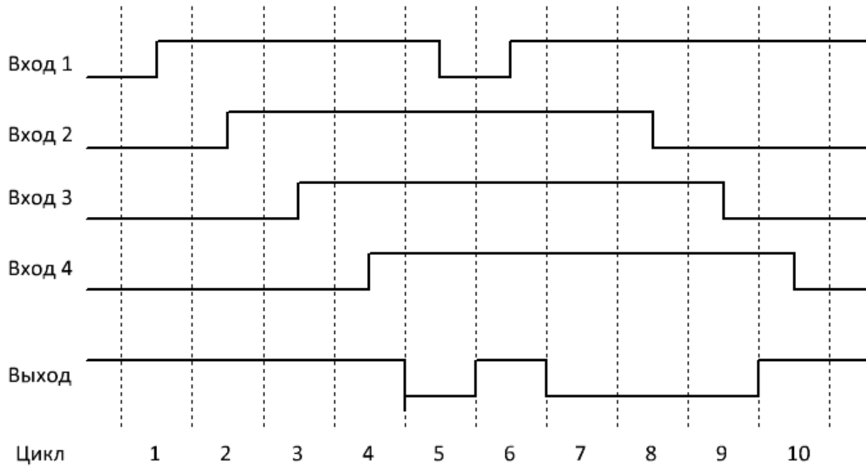
Рисунок 4.89 - Временная диаграмма
