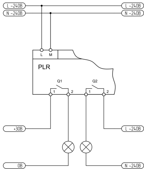
Рисунок 2.19 - Подключение релейного выхода
