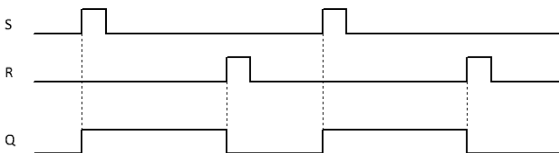
Рисунок 4.168 - Временная диаграмма
