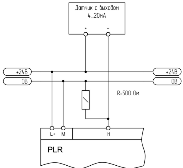
Рисунок 2.31 - Подключение к аналоговому датчику 4-20 мА
