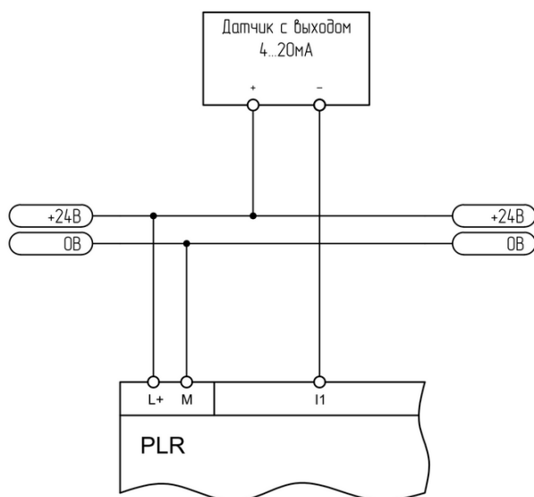
Рисунок 3.6 - Подключение к аналоговому датчику 4-20 мА
