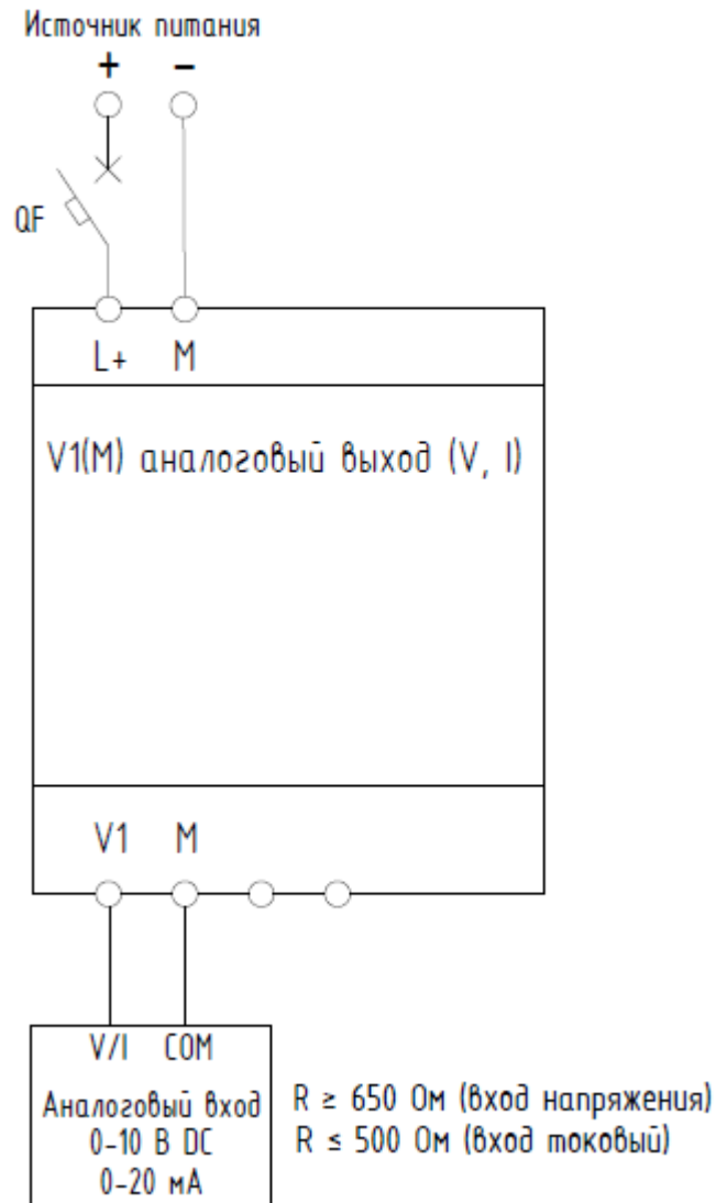
Рисунок 1.14 - Электрическая схема подключения модуля расширения
