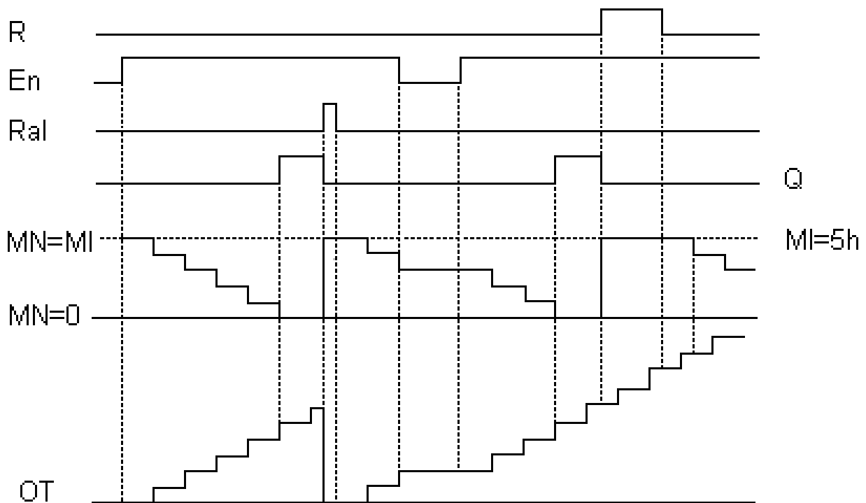
Рисунок 4.134 - Временная диаграмма
