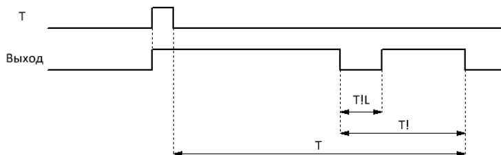
Рисунок 4.120 - Временная диаграмма
