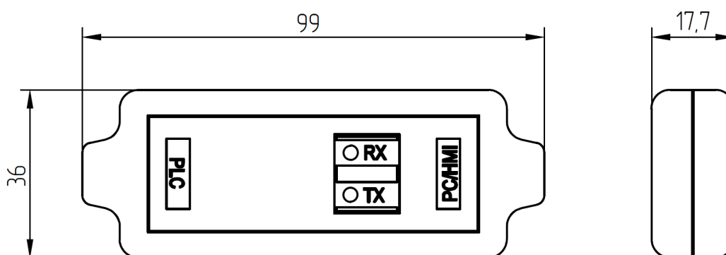
Рисунок 2.44 - Габаритные размеры кабеля
