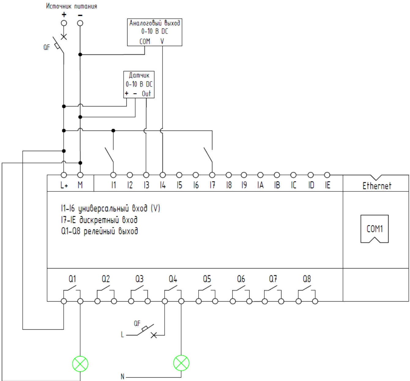
Рисунок 1.8 - Электрическая схема подключения модуля ЦПУ
