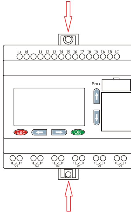
Рисунок 2.49 - Монтаж на поверхность
