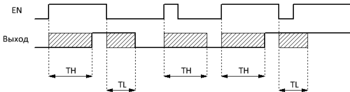
Рисунок 4.117 - Временная диаграмма
