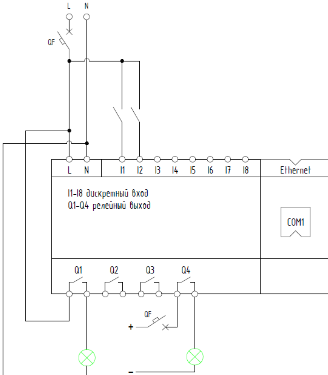
Рисунок 1.5 - Электрическая схема подключения модуля ЦПУ
