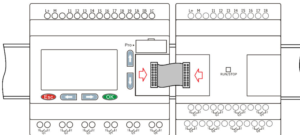
Рисунок 1.21 - Монтаж на DIN-рейку
