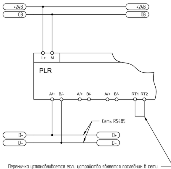
Рисунок 2.41 - Двухпроводное подключение
