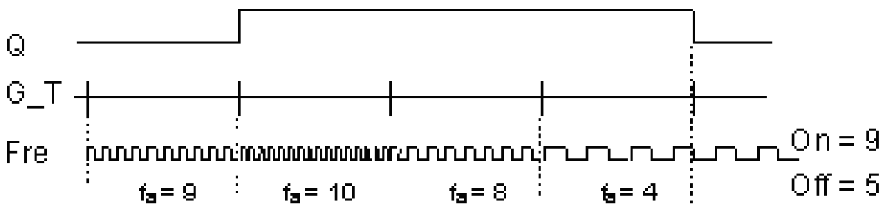
Рисунок 4.137 - Временная диаграмма
