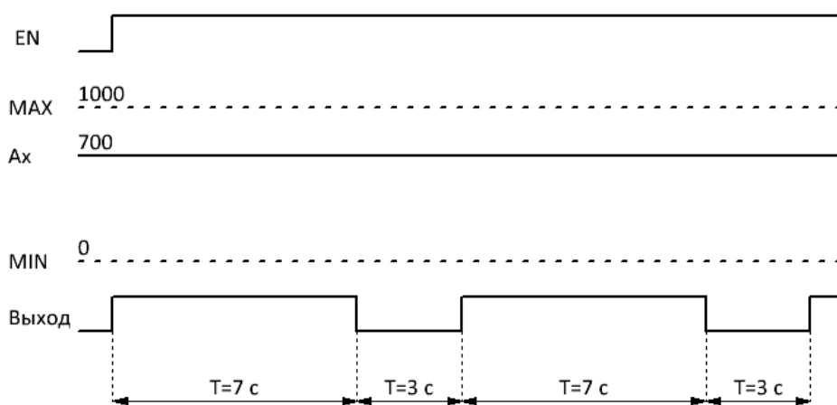
Рисунок 4.180 - Временная диаграмма
