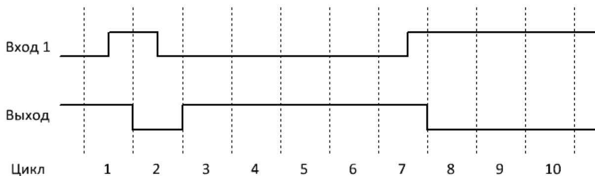
Рисунок 4.94 - Временная диаграмма
