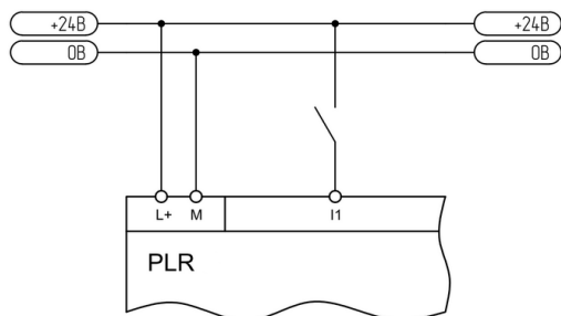
Рисунок 3.7 - Подключение к выходу "сухой контакт"
