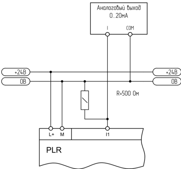
Рисунок 2.6 - Подключение к аналоговому выходу 0-20 мА
