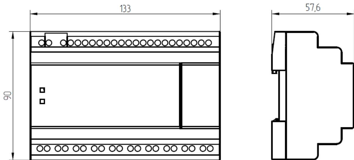
Рисунок 1.4 - Габаритные размеры модуля ЦПУ
