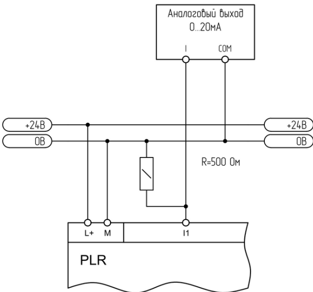
Рисунок 2.30 - Подключение к аналоговому выходу 0-20 мА
