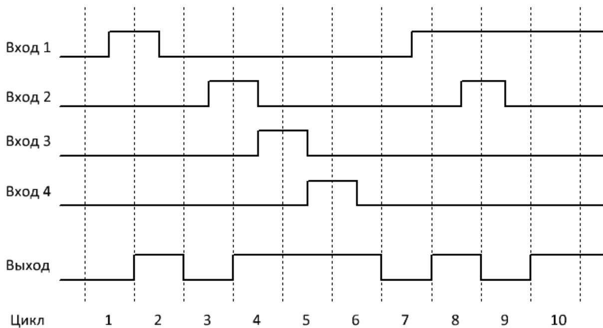
Рисунок 4.93 - Временная диаграмма
