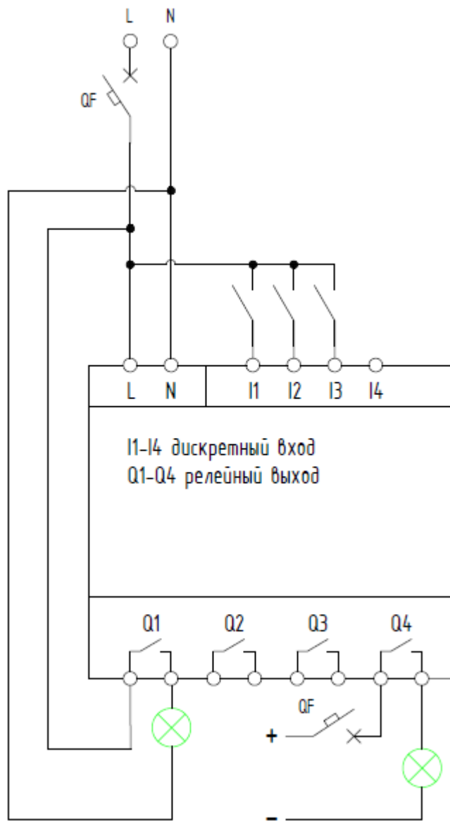
Рисунок 1.17 - Электрическая схема подключения модуля расширения
