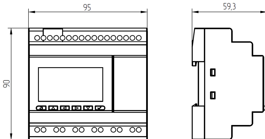
Рисунок 2.1 - Габаритные размеры модуля ЦПУ
