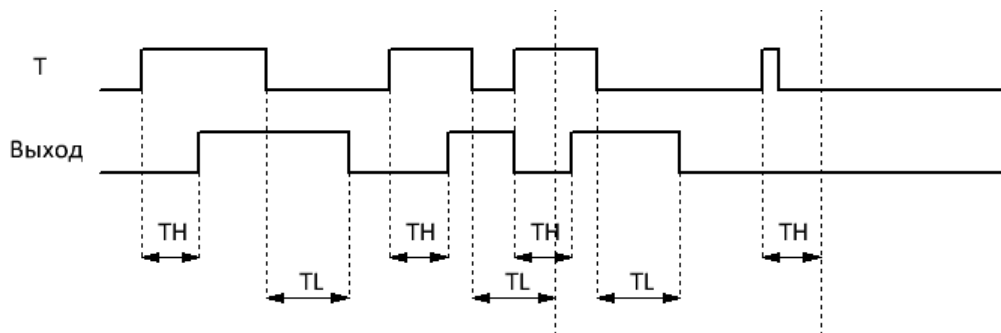
Рисунок 4.102 - Временная диаграмма
