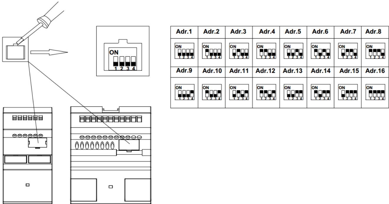
Рисунок 2.52 - Микропереключатели модуля расширения
