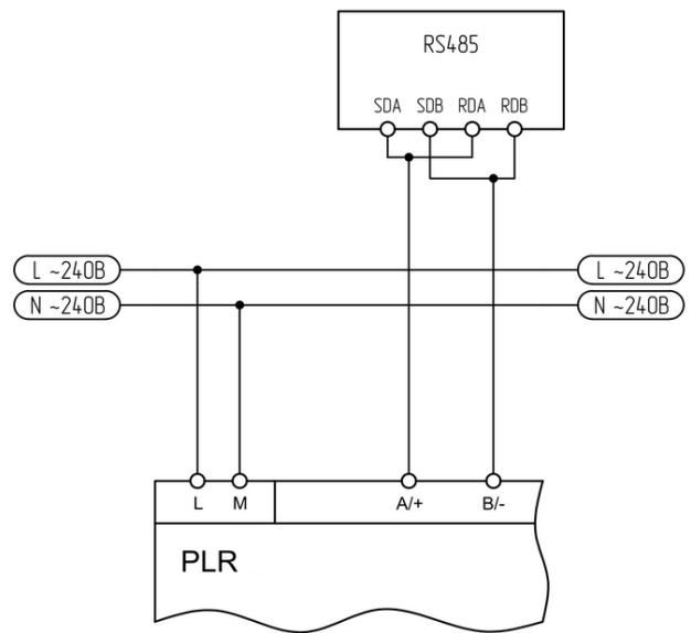
Рисунок 3.19 - Четырехпроводное подключение
