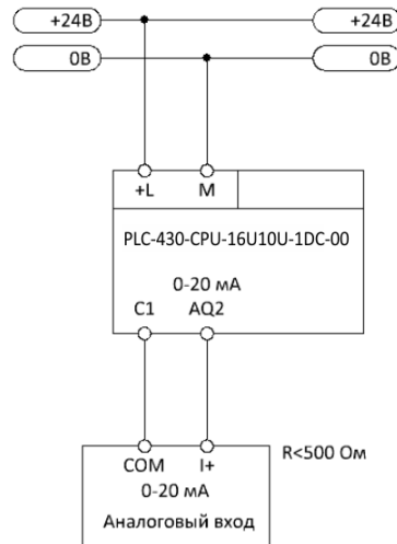
Рисунок 3.10 - Подключение к аналоговому входу 0-20 мА
