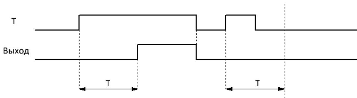
Рисунок 4.96 - Временная диаграмма
