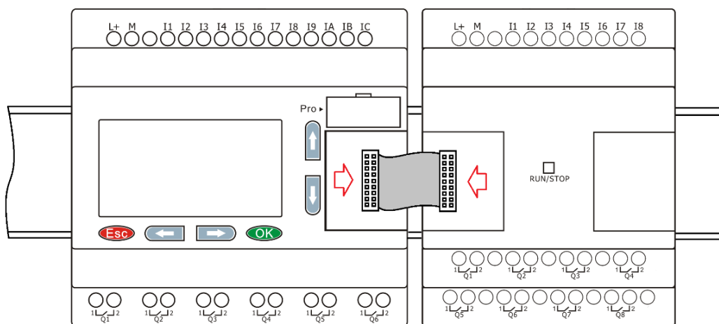
Рисунок 2.47 - Монтаж на DIN-рейку
