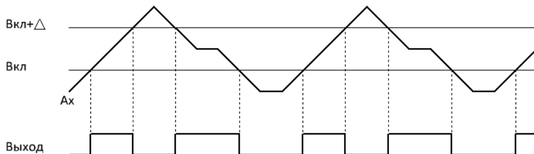
Рисунок 4.148 - Временная диаграмма для случая положительного диапазона ( \Delta > 0 )
