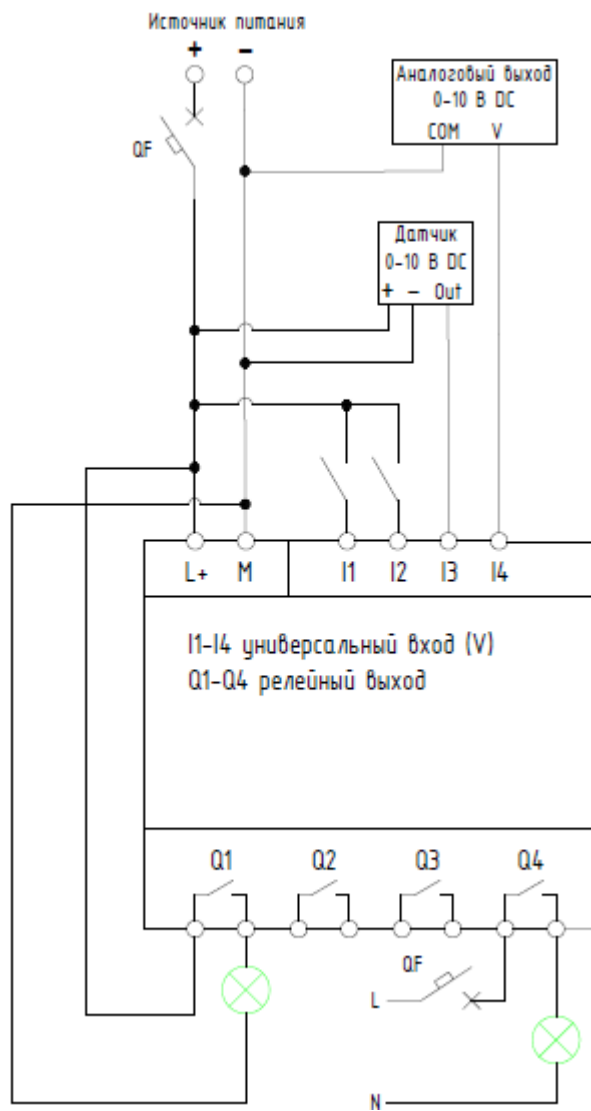
Рисунок 1.18 - Электрическая схема подключения модуля расширения
