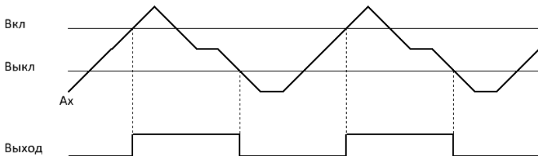
Рисунок 4.143 - Временная диаграмма для случая порога включения > порога выключения
