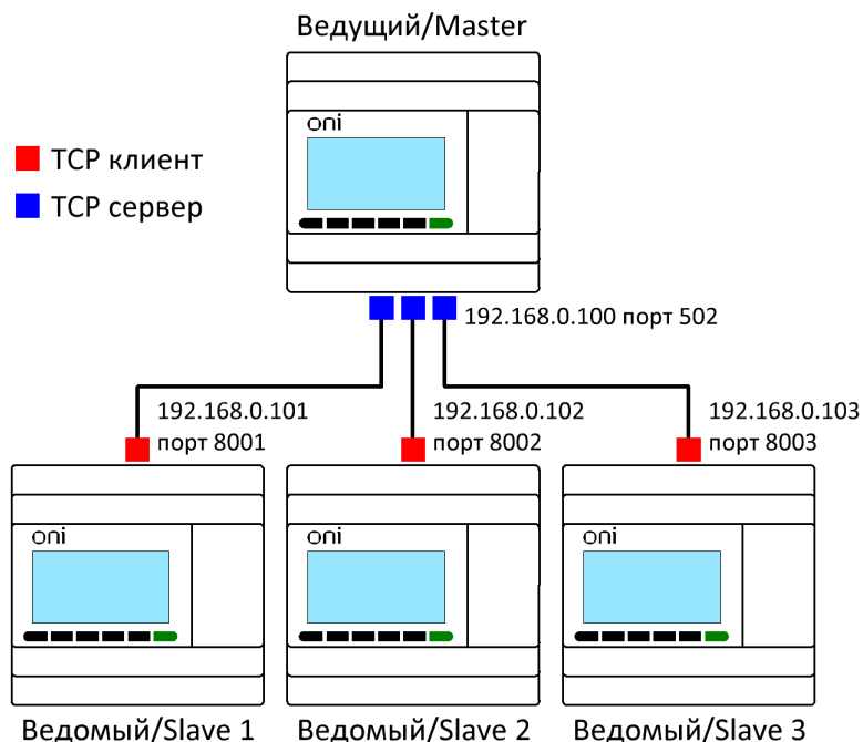
Рисунок 3.56 - Схема соединений
