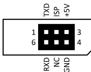
Рисунок 3.35 - Распиновка порта COM0
