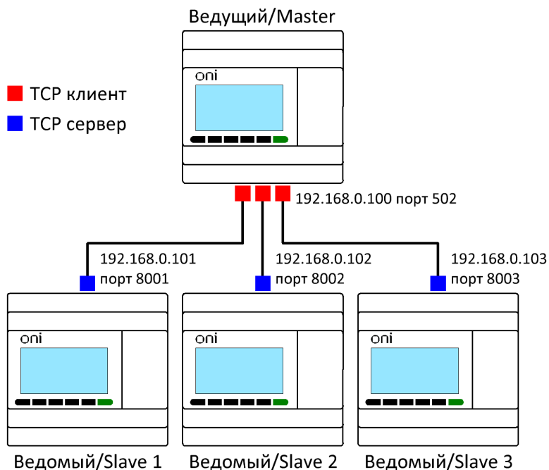
Рисунок 3.69 - Схема соединений
