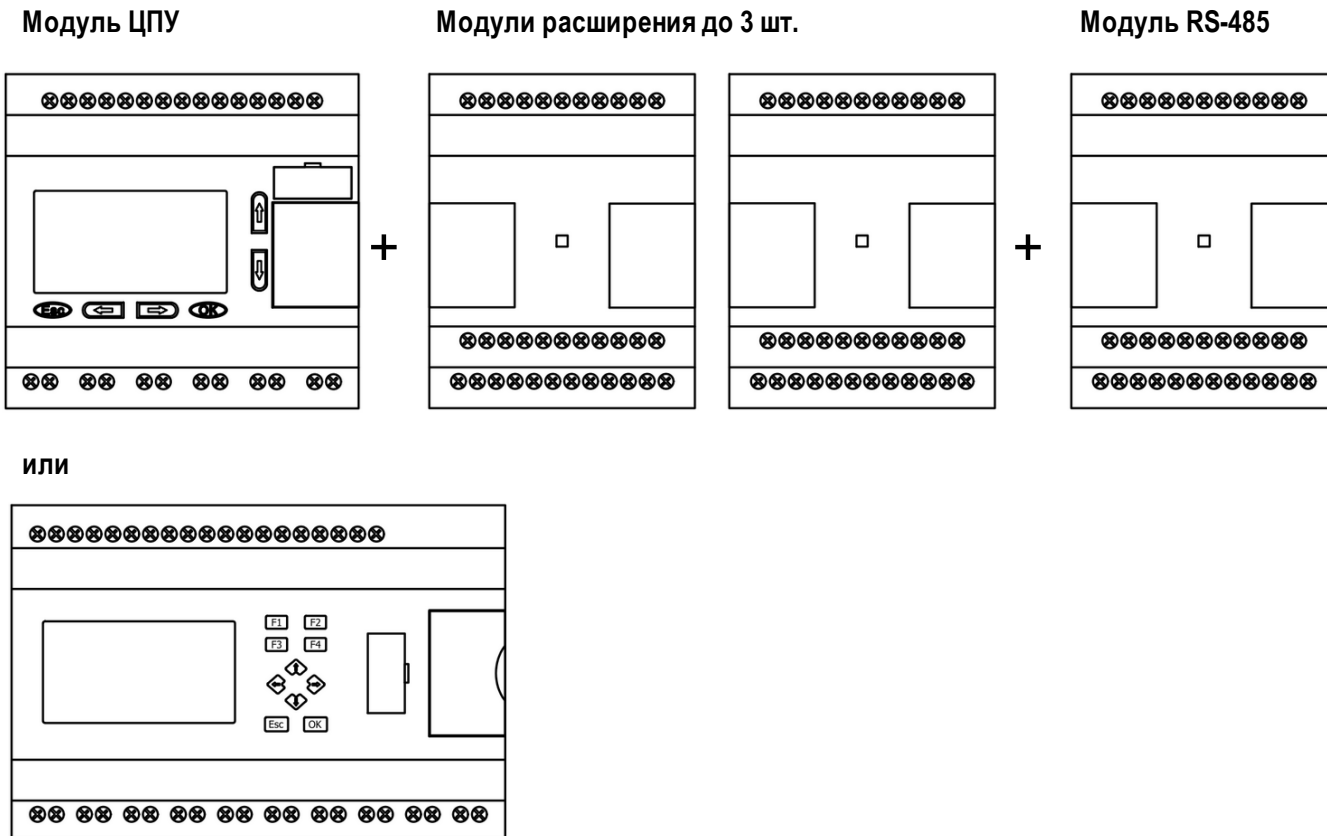
Рисунок 1.25 - Компоновка модулей расширения
