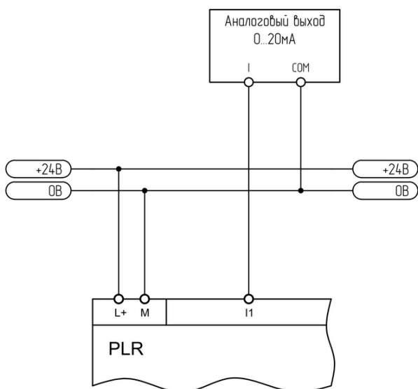
Рисунок 3.5 - Подключение к аналоговому выходу 0-20 мА
