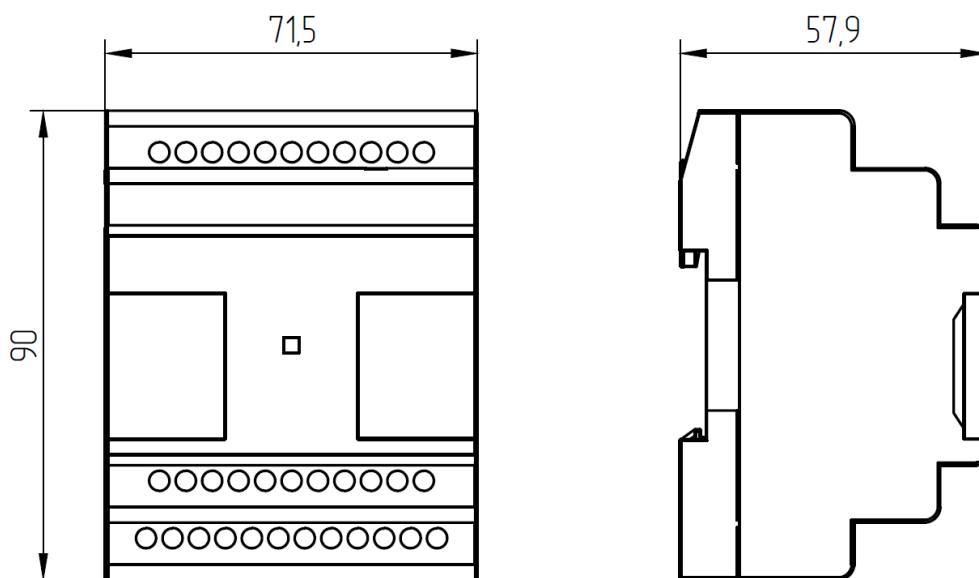
Рисунок 2.27 - Габаритные размеры модуля расширения
