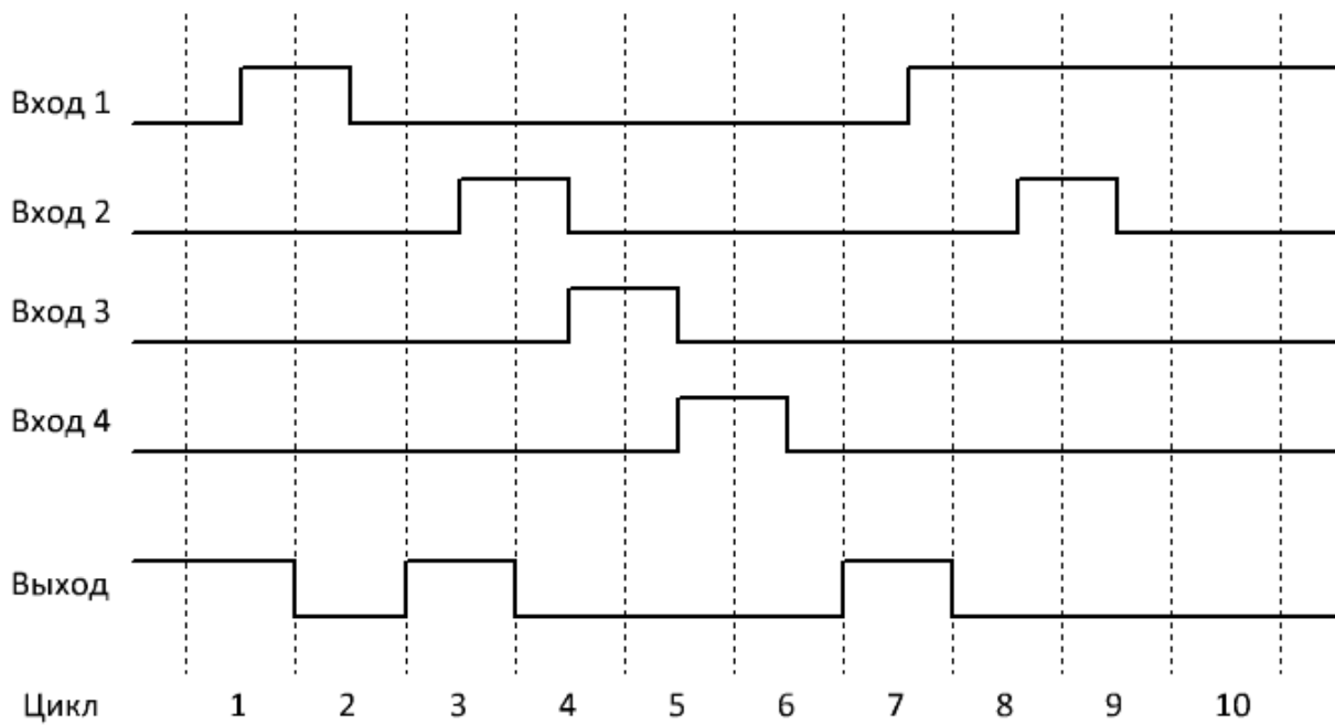
Рисунок 4.92 - Временная диаграмма
