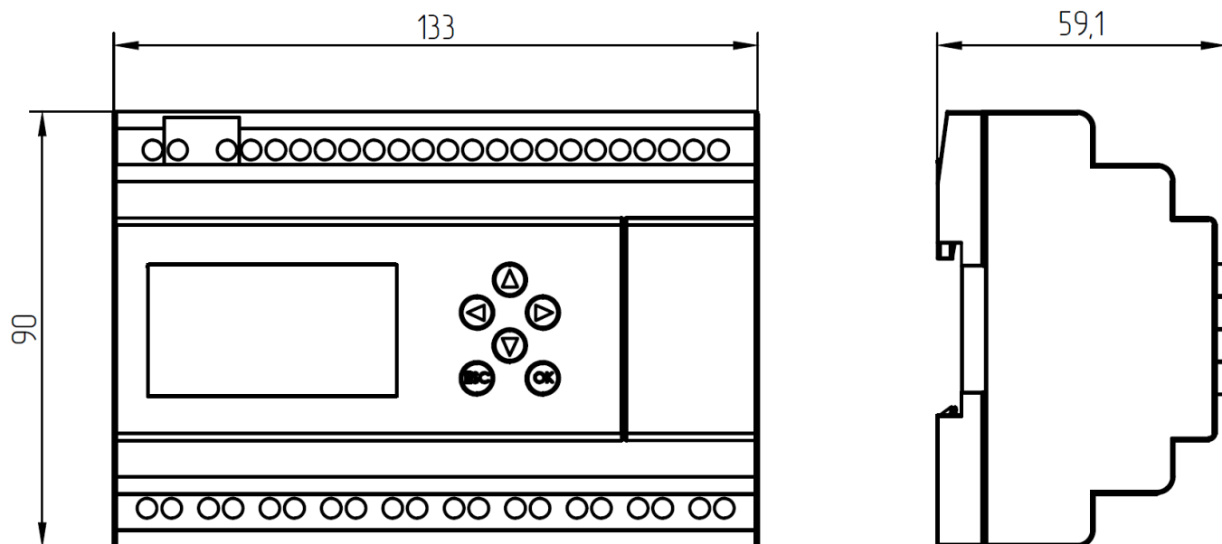
Рисунок 3.2 - Габаритные размеры модуля ЦПУ
