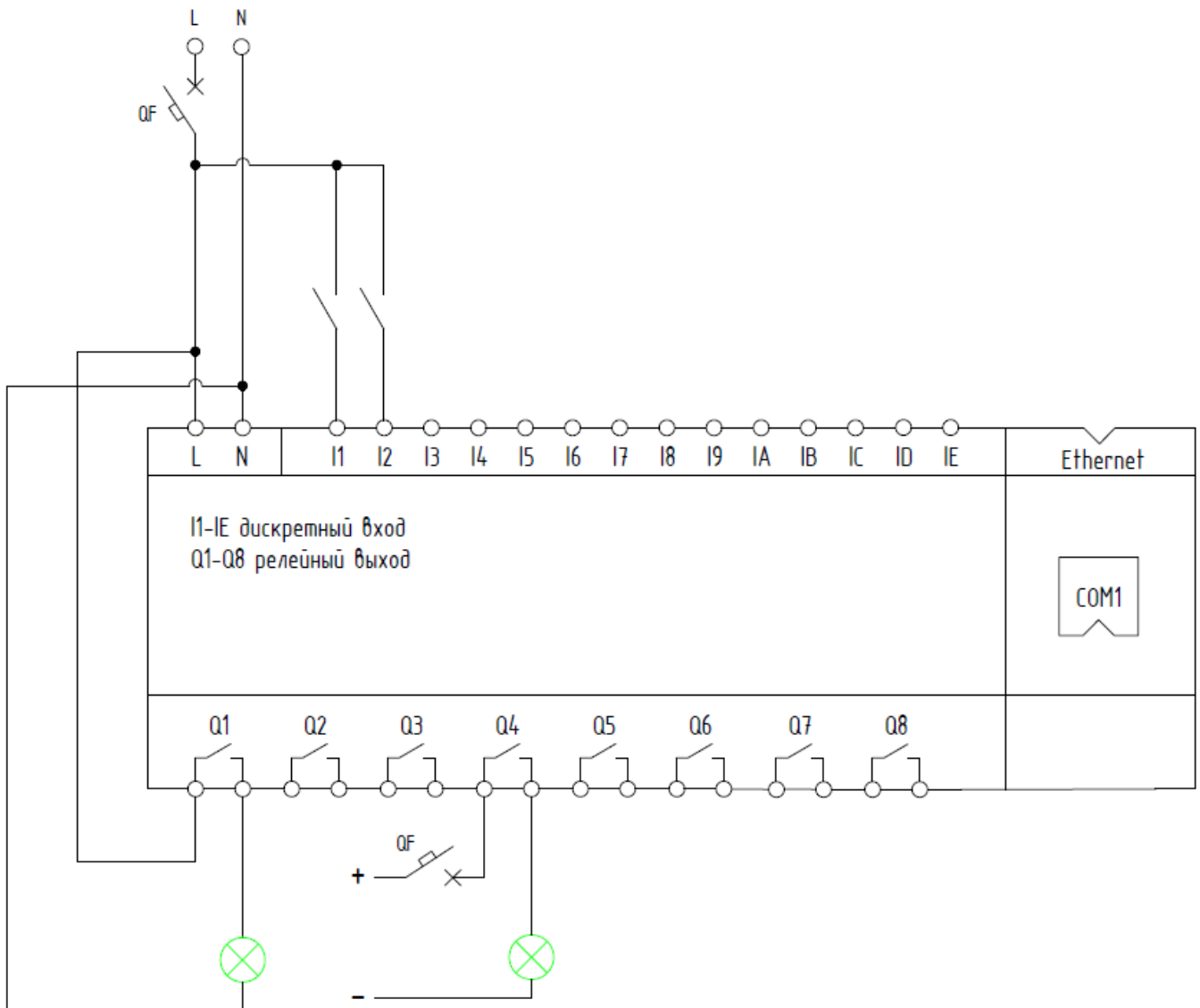
Рисунок 1.7 - Электрическая схема подключения модуля ЦПУ
