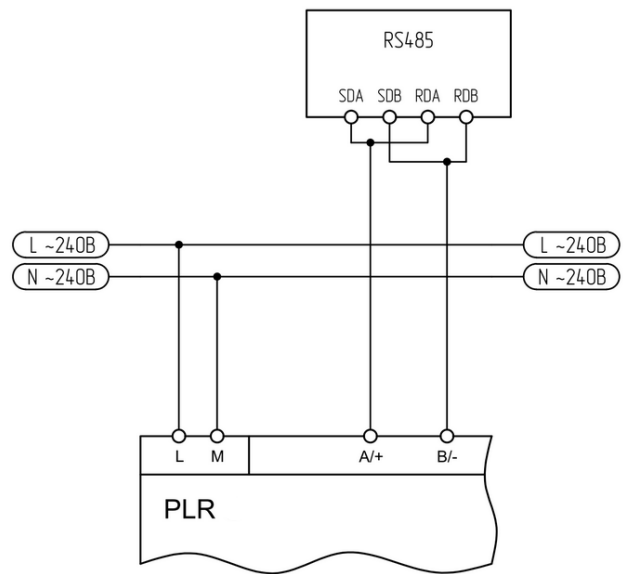
Рисунок 2.21 - Четырехпроводное подключение
