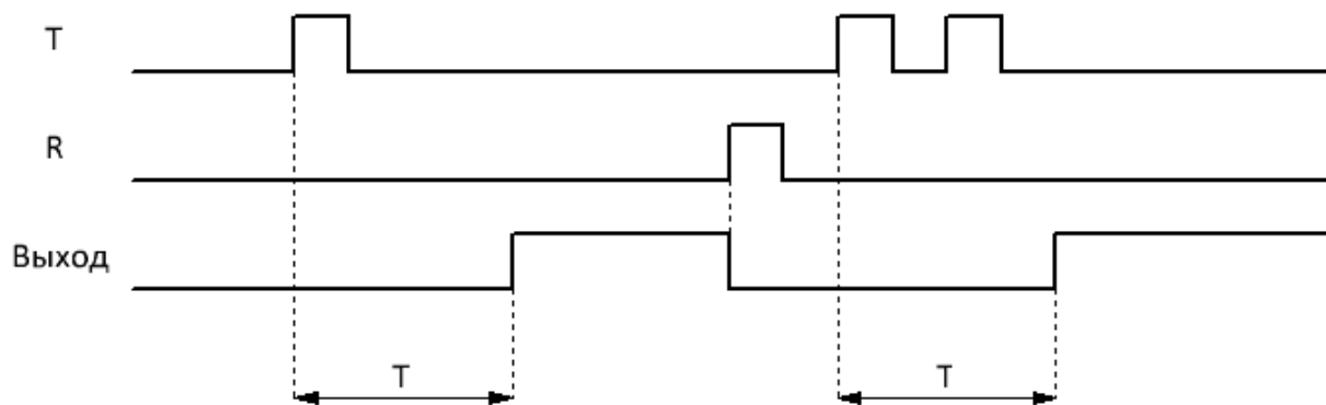
Рисунок 4.105 - Временная диаграмма
