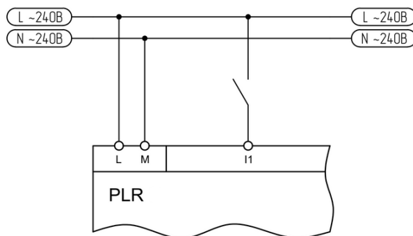
Рисунок 3.16 - Подключение к выходу "сухой контакт"
