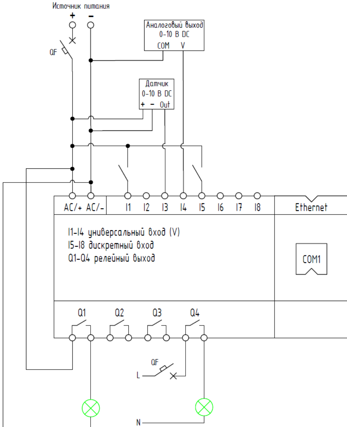
Рисунок 1.6 - Электрическая схема подключения модуля ЦПУ
