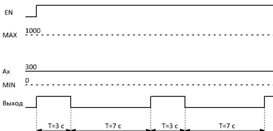
Рисунок 4.181 - Временная диаграмма
