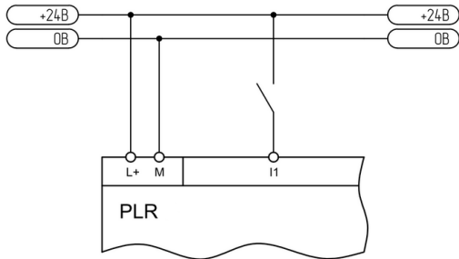
Рисунок 2.35 - Подключение к выходу "сухой контакт"
