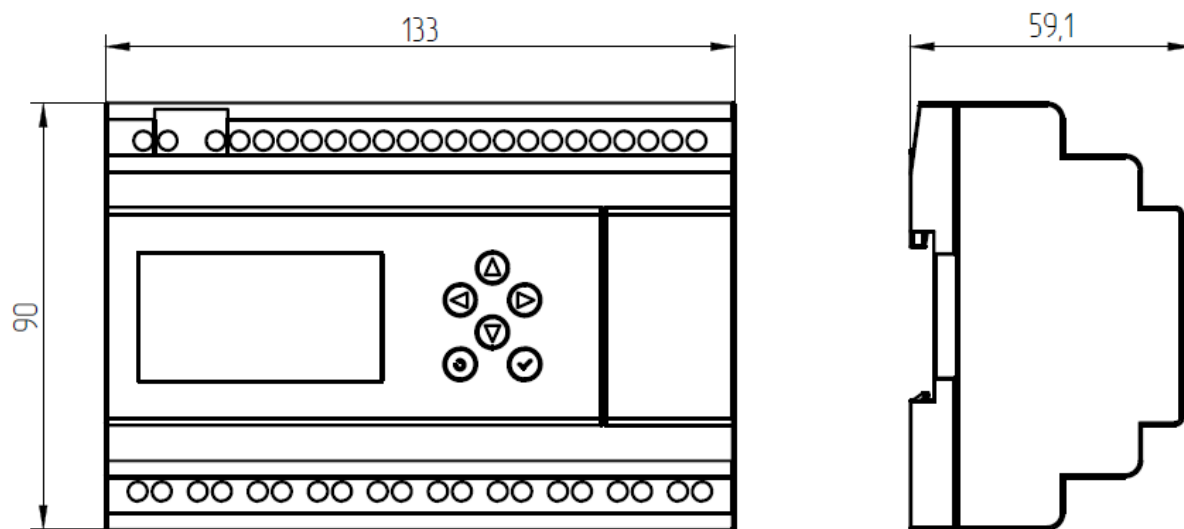
Рисунок 1.3 - Габаритные размеры модуля ЦПУ
