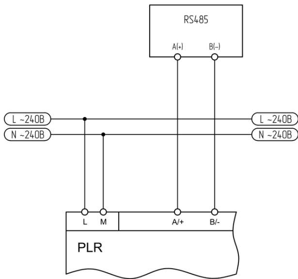
Рисунок 2.20 - Двухпроводное подключение
