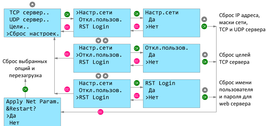
Рисунок 3.23 - Системное меню сети Ethernet
