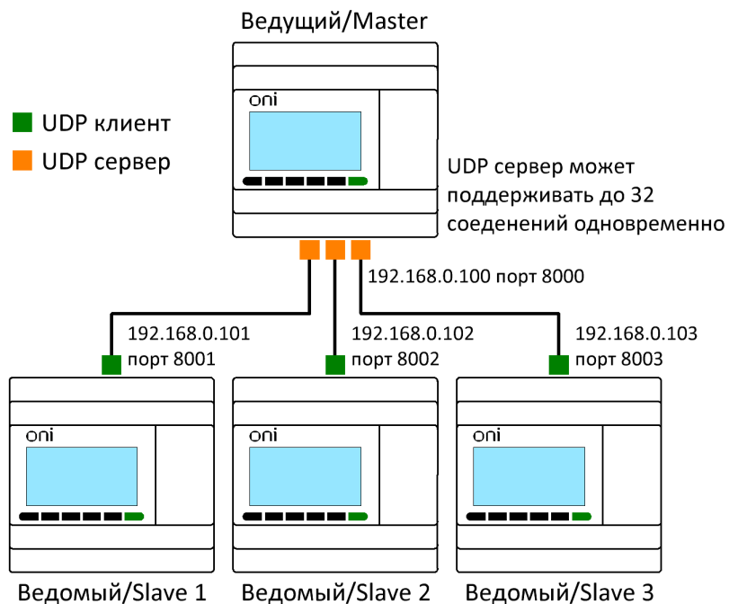
Рисунок 3.85 - Схема соединений
