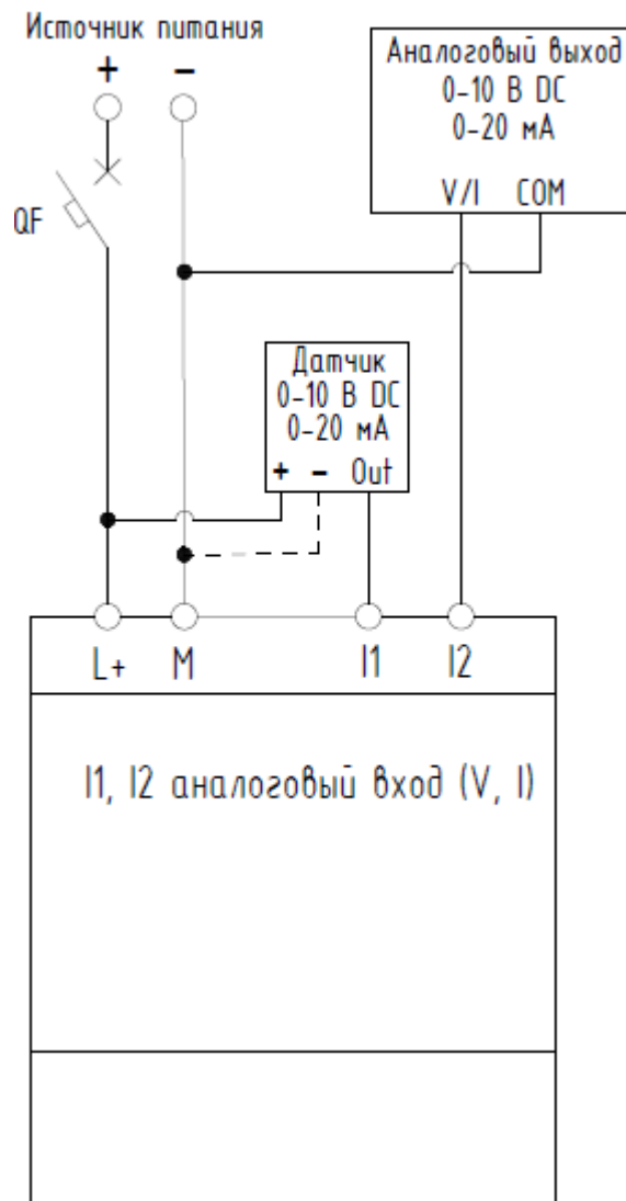
Рисунок 1.16 - Электрическая схема подключения модуля расширения
