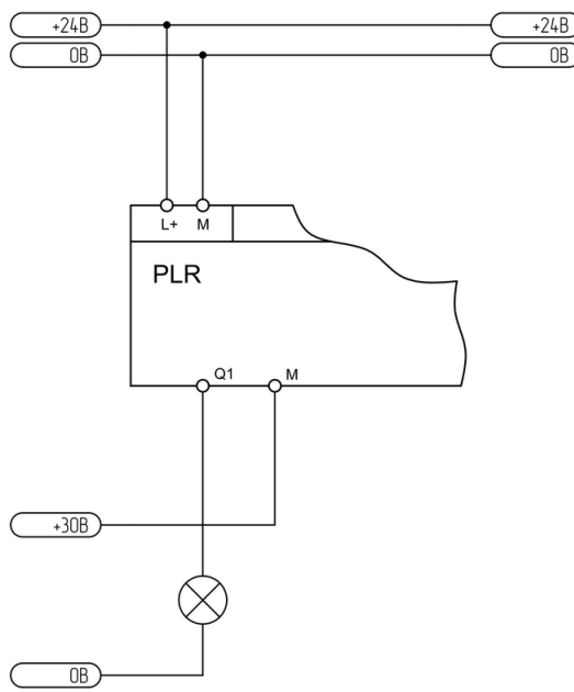
Рисунок 2.15 - Подключение транзисторного выхода
