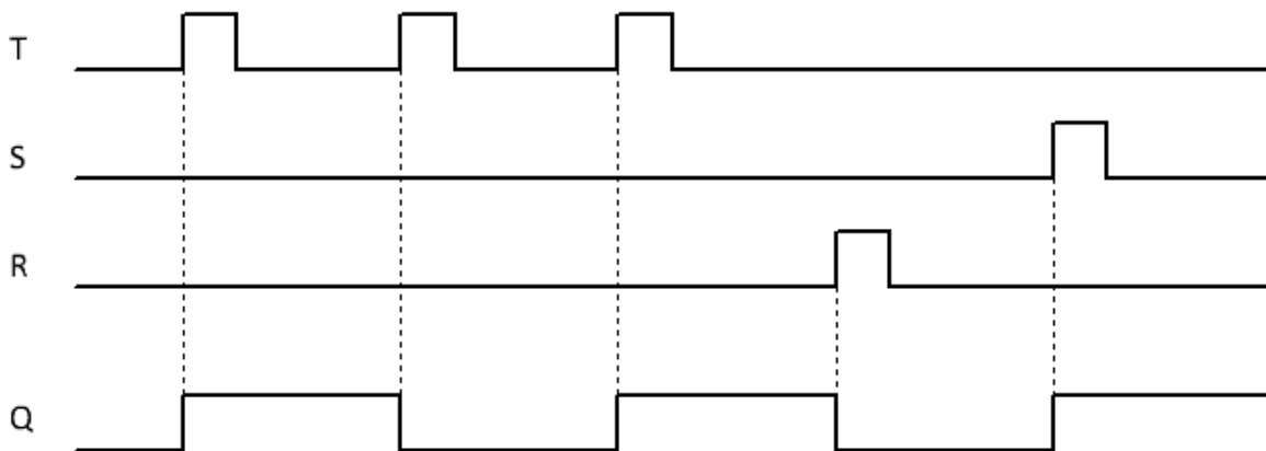
Рисунок 4.169 - Временная диаграмма
