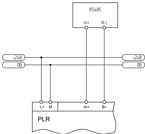
Рисунок 3.14 - Двухпроводное подключение
