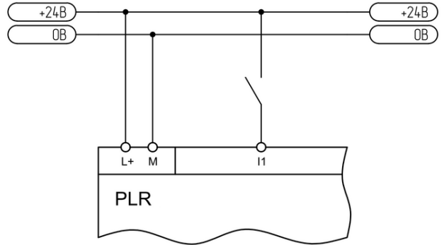
Рисунок 2.29 - Подключение к выходу "сухой контакт"
