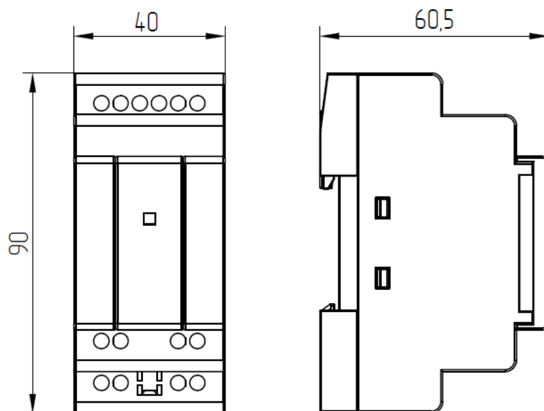
Рисунок 2.26 - Габаритные размеры модуля расширения
