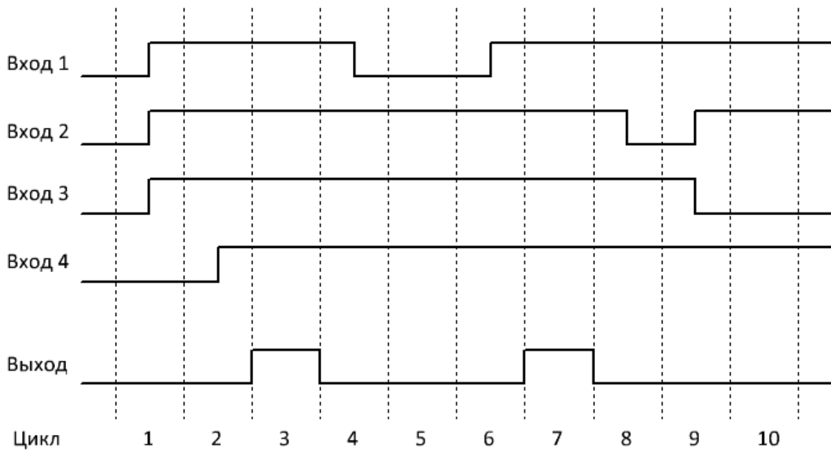
Рисунок 4.88 - Временная диаграмма
