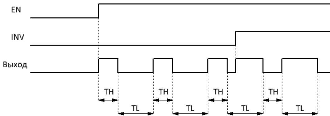
Рисунок 4.114 - Временная диаграмма
