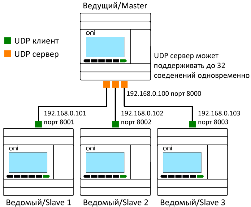
Рисунок 1.75 - Схема соединений
