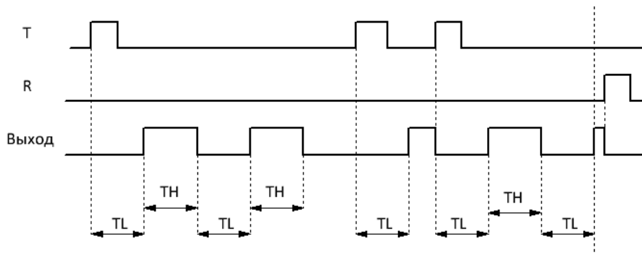
Рисунок 4.111 - Временная диаграмма
