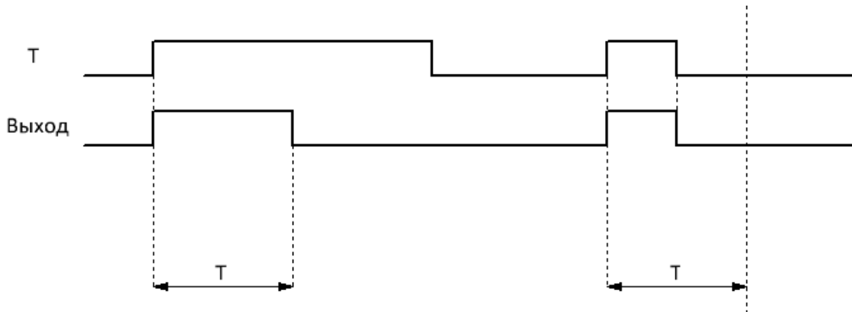
Рисунок 4.108 - Временная диаграмма
