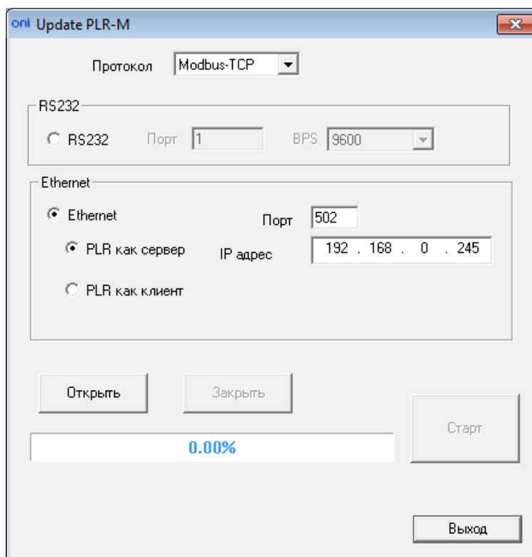
Рисунок 1.27 - Обновление прошивки
