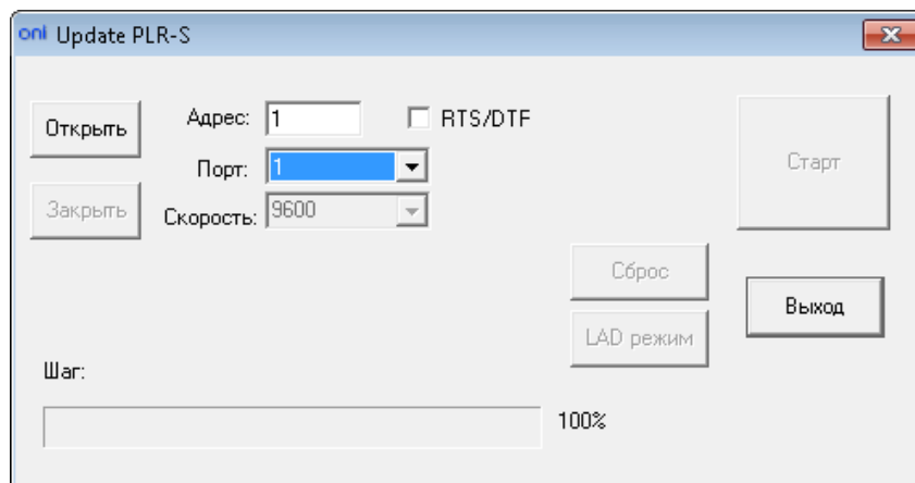
Рисунок 2.57 - Обновление прошивки
