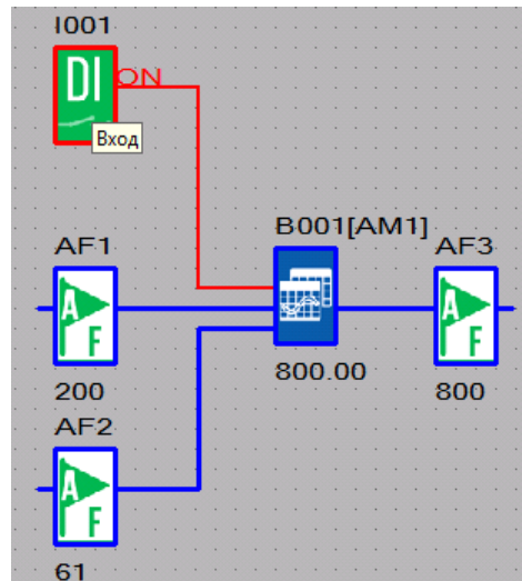
Рисунок 4.216 - Программа
