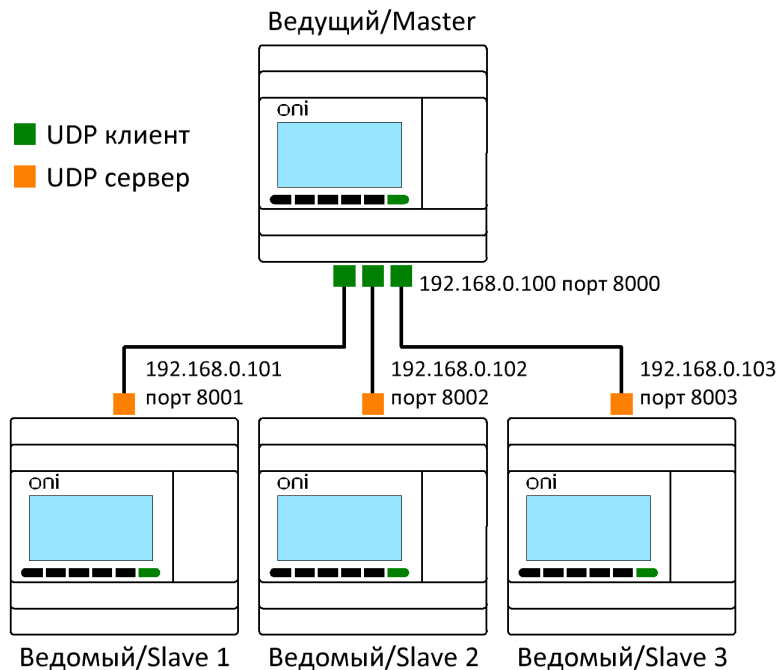
Рисунок 1.88 - Схема соединений
