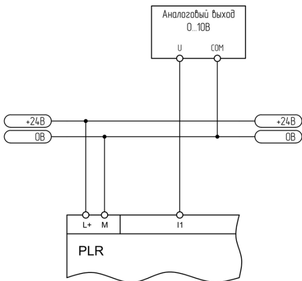
Рисунок 3.3 - Подключение к аналоговому выходу 0-10 В
