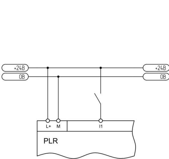
Рисунок 2.10 - Подключение к выходу "сухой контакт"
