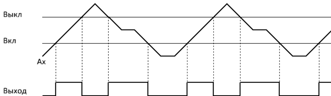
Рисунок 4.144 - Временная диаграмма для случая порога включения < порога выключения
