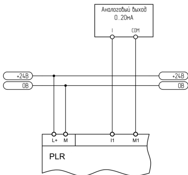
Рисунок 2.32 - Подключение к аналоговому выходу 0-20 мА
