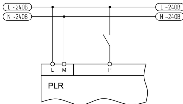
Рисунок 2.42 - Подключение к выходу "сухой контакт"
