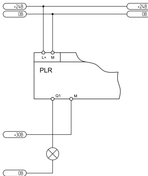
Рисунок 2.40 - Подключение транзисторного выхода
