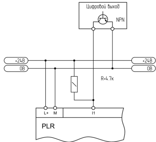
Рисунок 2.36 - Подключение к выходу "открытый коллектор"
