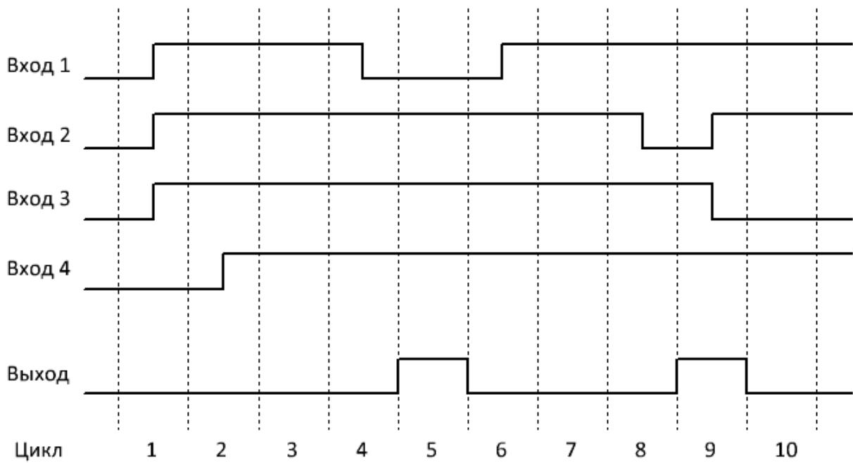
Рисунок 4.90 - Временная диаграмма
