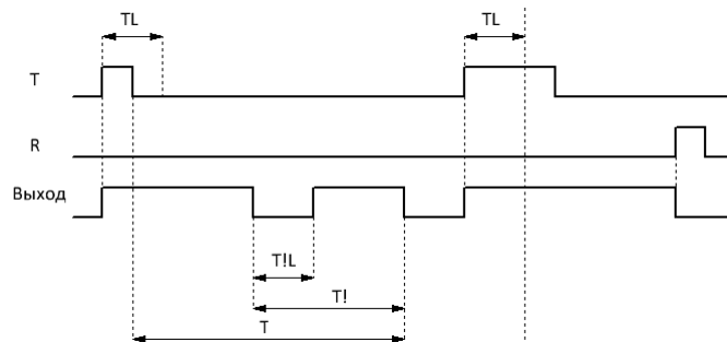
Рисунок 4.123 - Временная диаграмма
