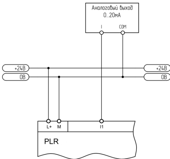
Рисунок 2.8 - Подключение к аналоговому выходу 0-20 мА
