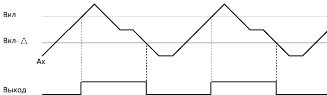
Рисунок 4.147 - Временная диаграмма для случая отрицательного диапазона ( \Delta < 0 )
