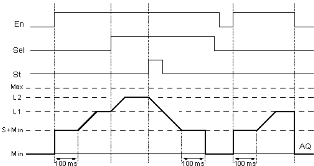
Рисунок 4.183 - Временная диаграмма
