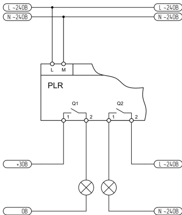
Рисунок 2.43 - Подключение релейного выхода
