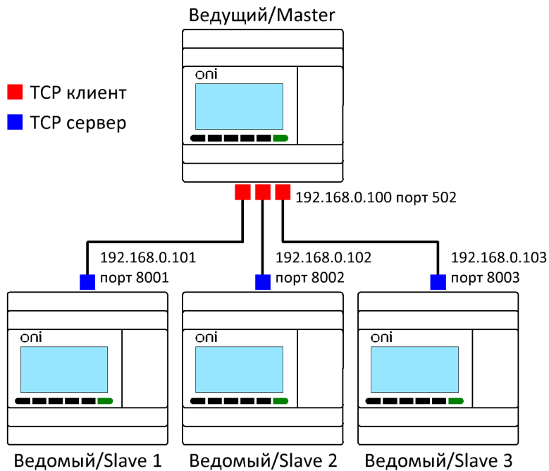
Рисунок 1.59 - Схема соединений
