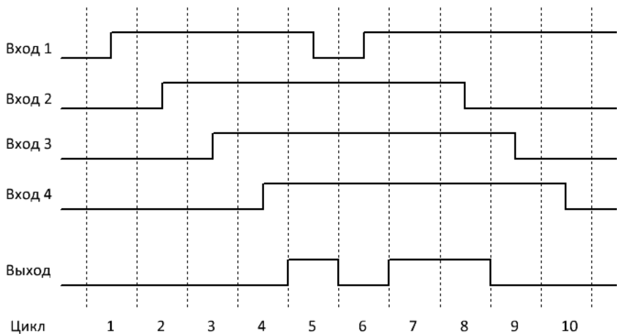
Рисунок 4.87 - Временная диаграмма
