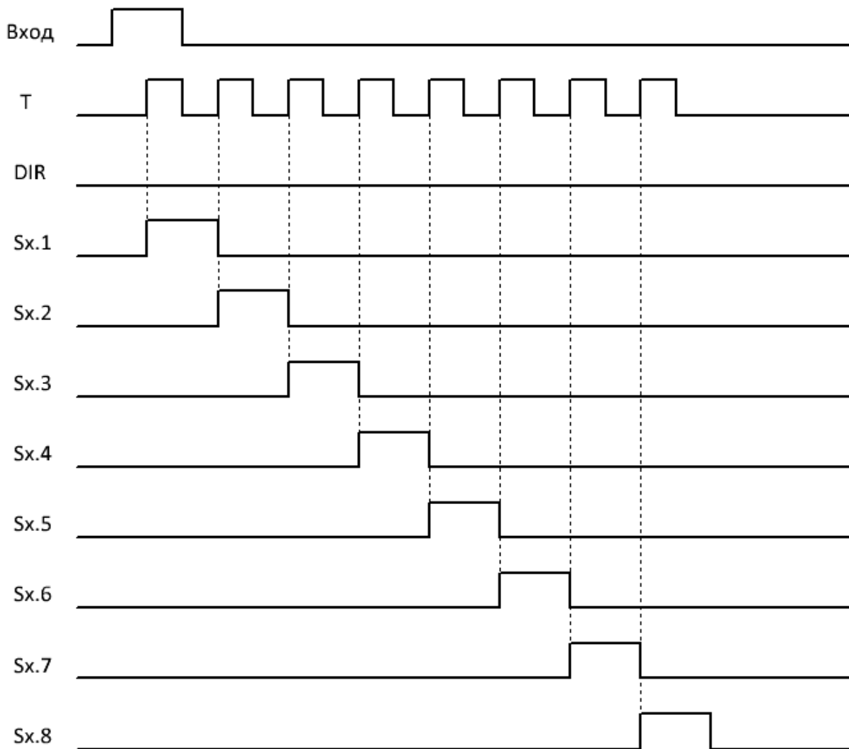
Рисунок 4.170 - Временная диаграмма
