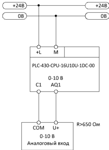
Рисунок 3.9 - Подключение к аналоговому входу 0-10 В
