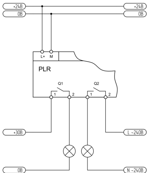
Рисунок 2.39 - Подключение релейного выхода
