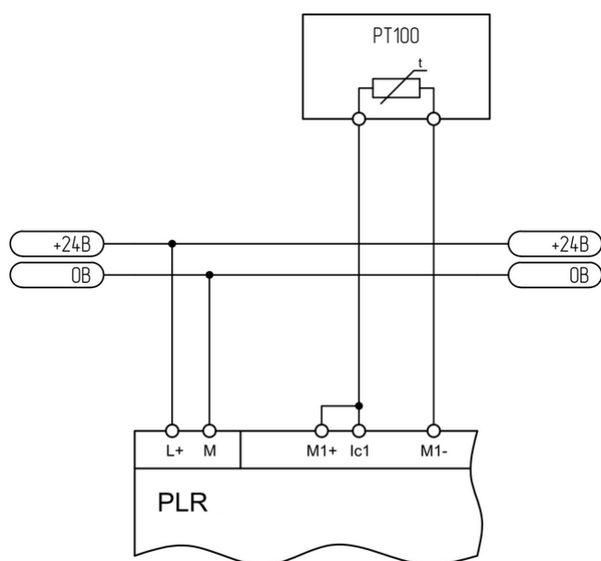
Рисунок 2.34 - Подключение термосопротивления 2-проводное
