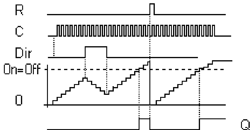
Рисунок 4.131 - Временная диаграмма
