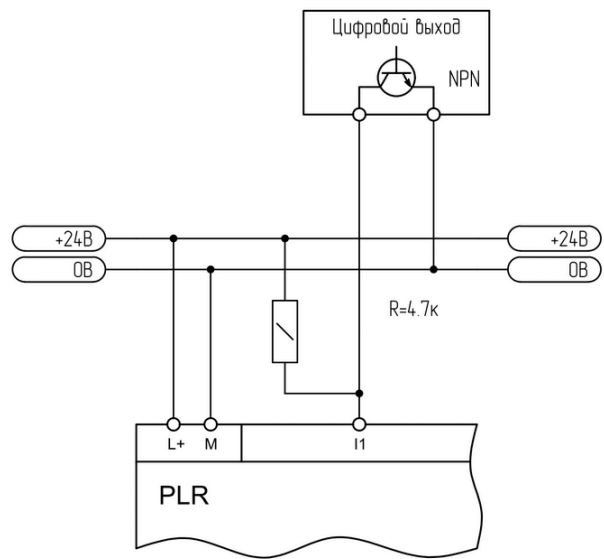
Рисунок 2.11 - Подключение к выходу "открытый коллектор"
