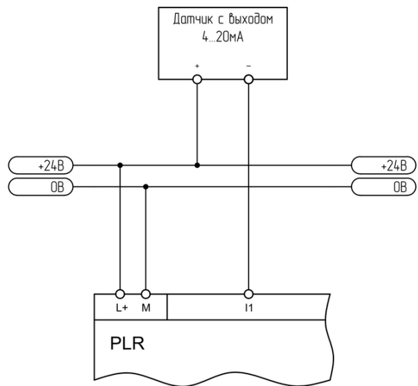
Рисунок 2.9 - Подключение к аналоговому датчику 4-20 мА
