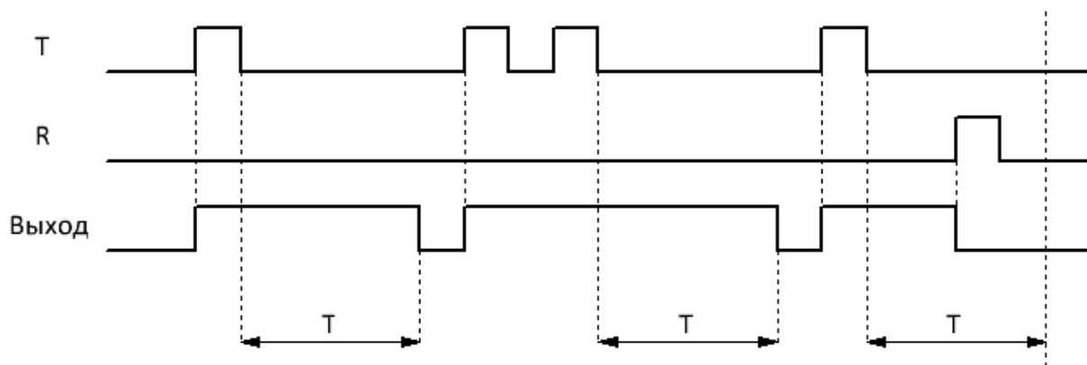
Рисунок 4.99 - Временная диаграмма
