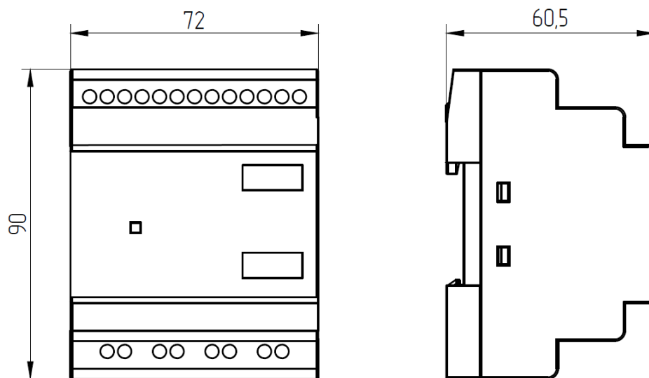
Рисунок 2.3 - Габаритные размеры модуля ЦПУ
