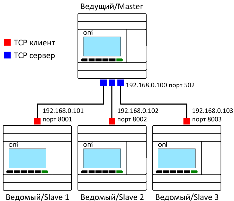
Рисунок 1.46 - Схема соединений
