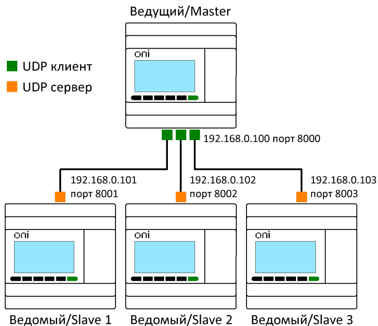
Рисунок 3.98 - Схема соединений
