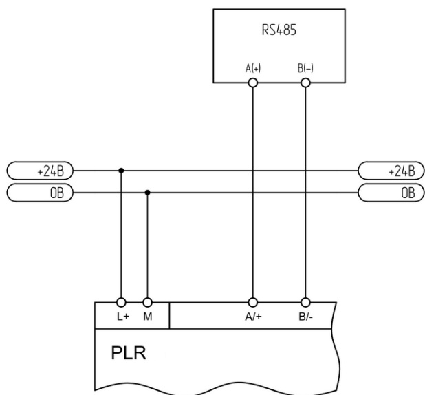
Рисунок 2.16 - Двухпроводное подключение
