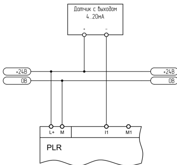
Рисунок 2.33 - Подключение к аналоговому датчику 4-20 мА
