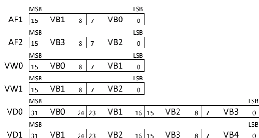
Рисунок 4.81 - Организация структуры памяти
