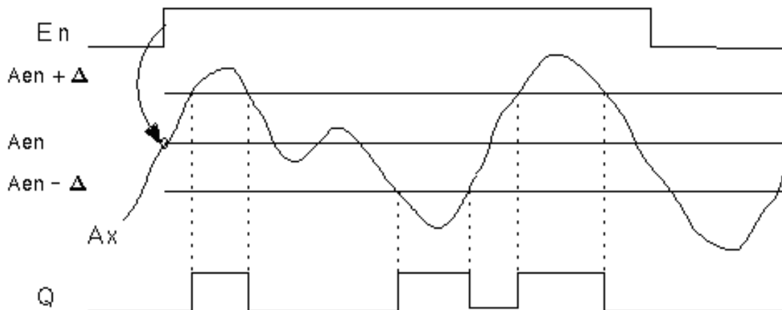
Рисунок 4.151 - Временная диаграмма
