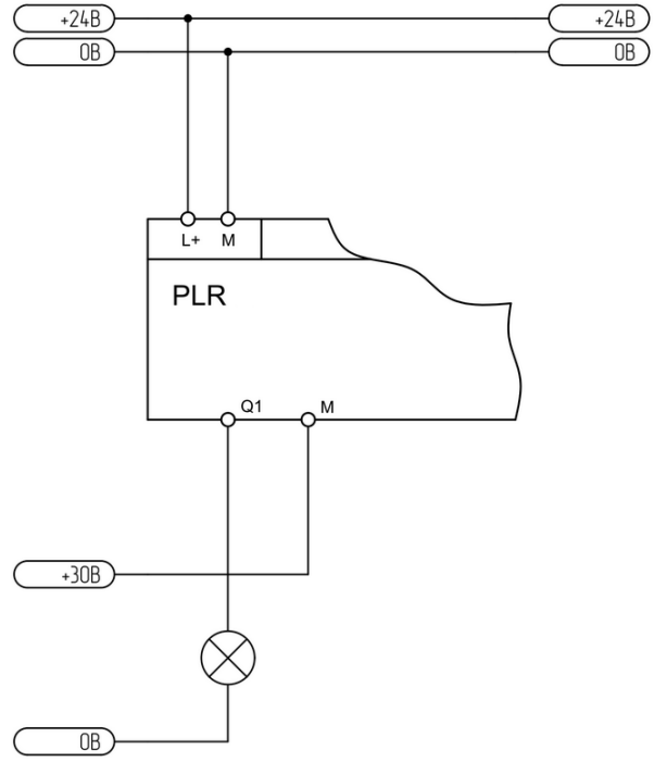
Рисунок 3.12 - Подключение транзисторного выхода
