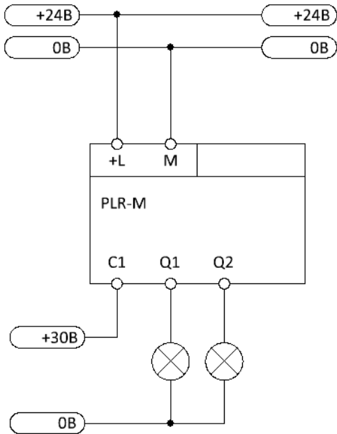
Рисунок 3.13 - Подключение транзисторного выхода
