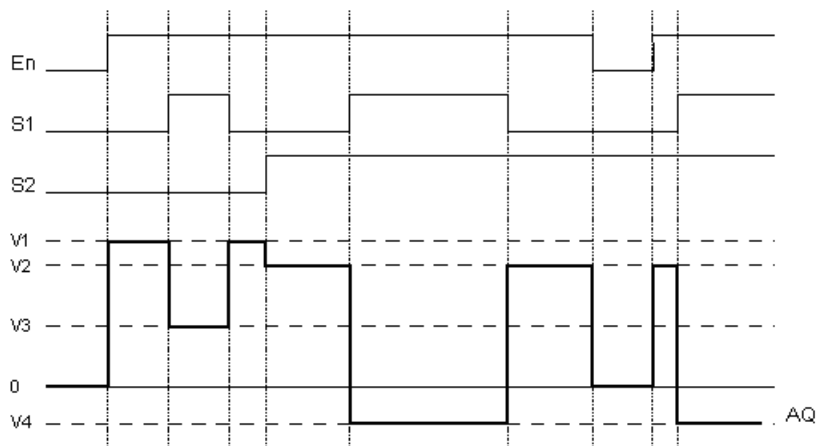
Рисунок 4.154 - Временная диаграмма
