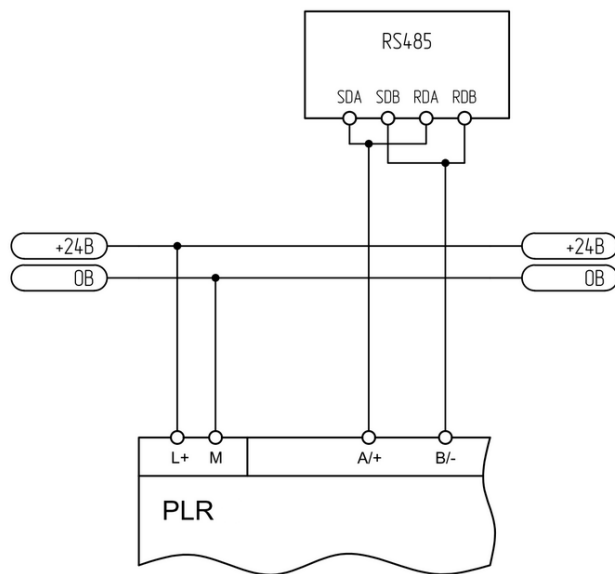
Рисунок 3.15 - Четырехпроводное подключение
