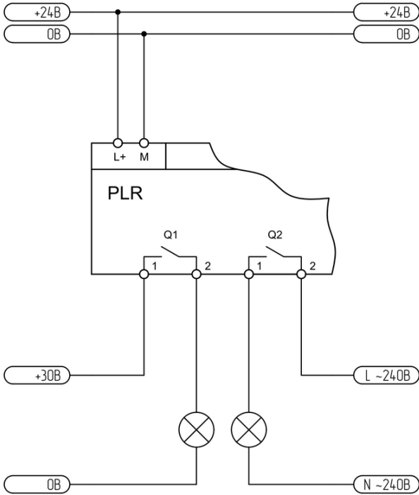
Рисунок 3.11 - Подключение релейного выхода
