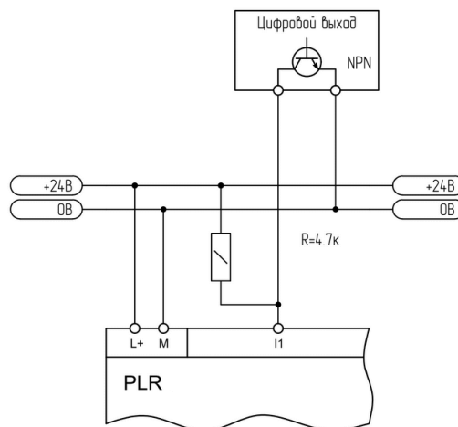
Рисунок 3.8 - Подключение к выходу "открытый коллектор"
