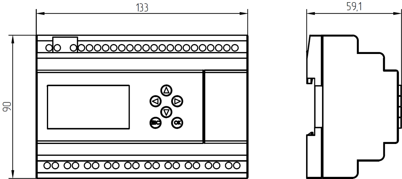
Рисунок 2.2 - Габаритные размеры модуля ЦПУ
