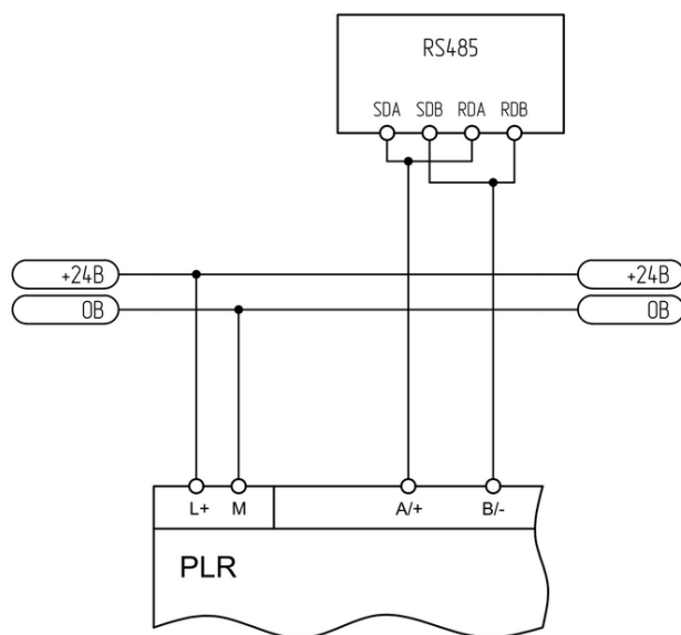
Рисунок 2.17 - Четырехпроводное подключение
