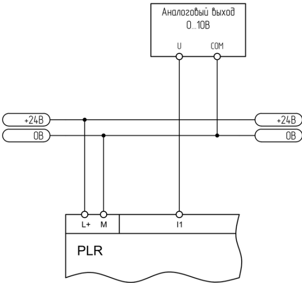
Рисунок 2.28 - Подключение к аналоговому выходу 0-10 В
