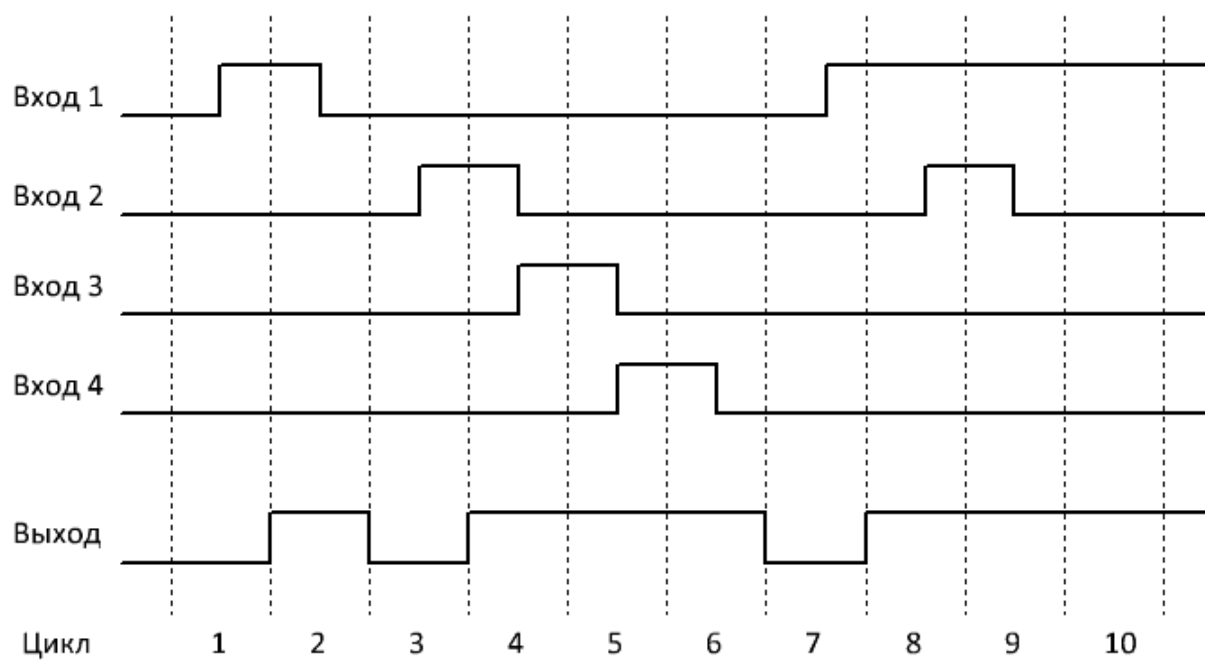
Рисунок 4.91 - Временная диаграмма
