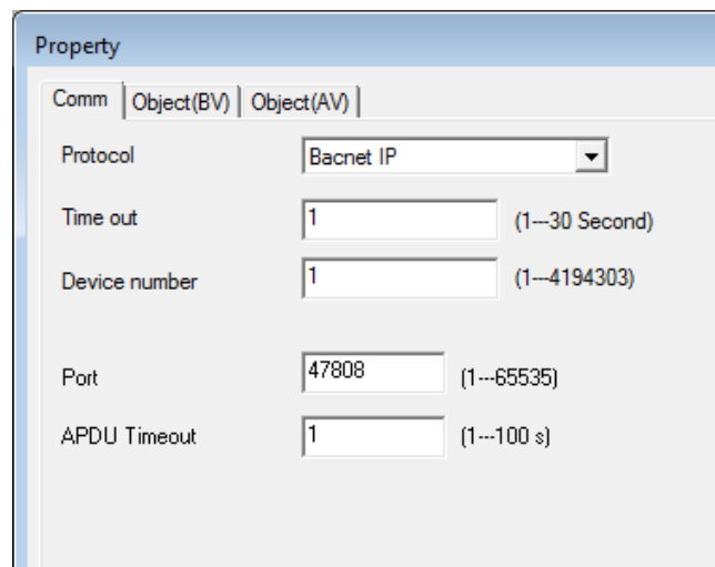
Рисунок 4.61 - Вкладка "Comm"
