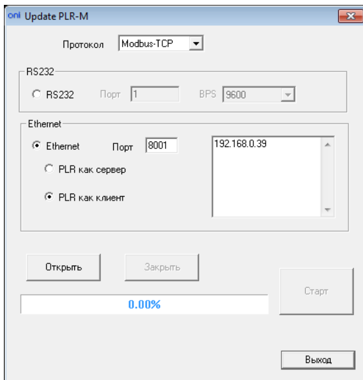
Рисунок 1.28 - Обновление прошивки
