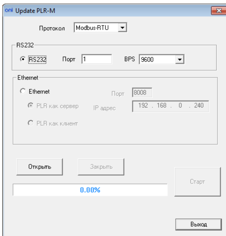
Рисунок 3.36 - Обновление прошивки
