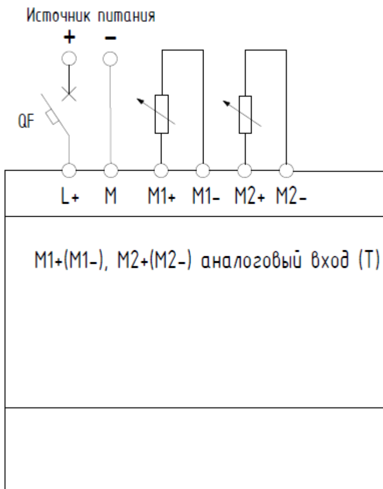
Рисунок 1.15 - Электрическая схема подключения модуля расширения
