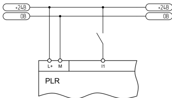
Рисунок 3.4 - Подключение к выходу "сухой контакт"
