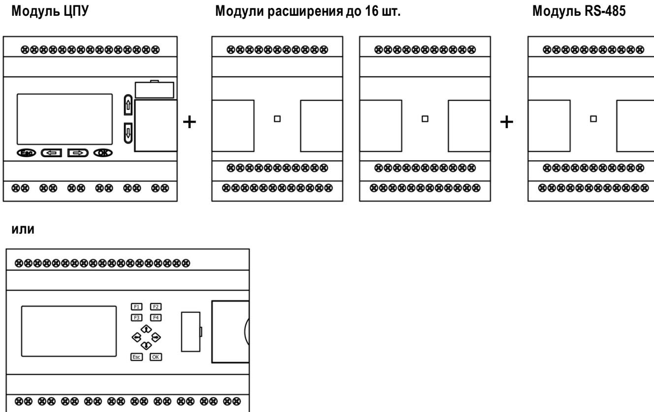
Рисунок 2.51 - Компоновка модулей расширения
