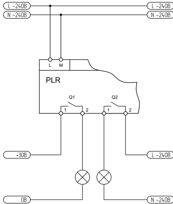
Рисунок 3.17 - Подключение релейного выхода
