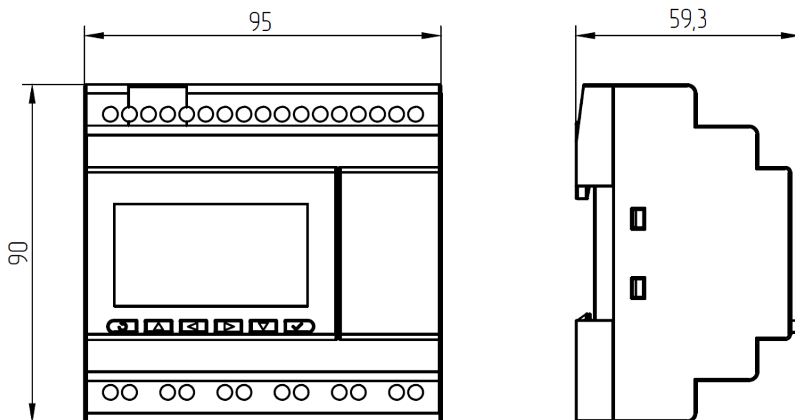
Рисунок 3.1 - Габаритные размеры модуля ЦПУ
