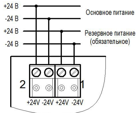
Рисунок 9 – Подключение питания ППК
